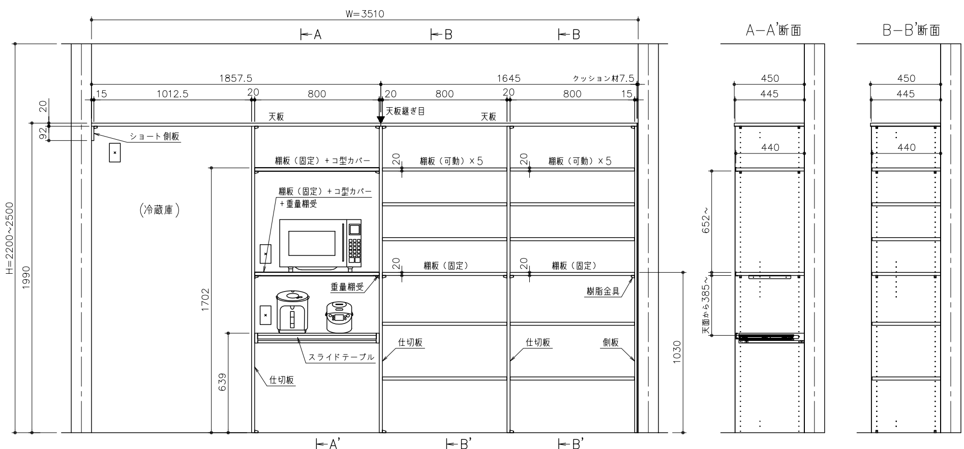
[正面図]
